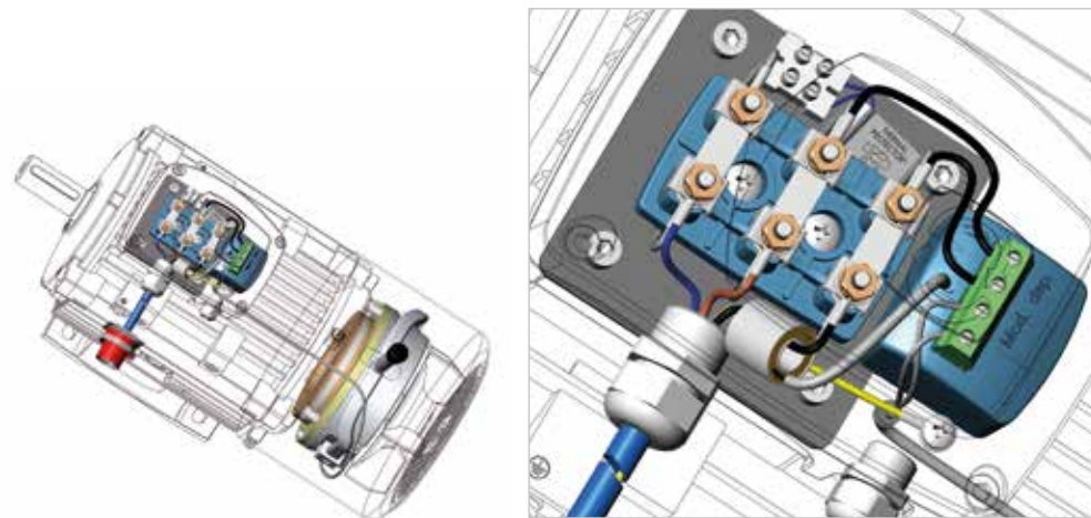
ATDC \triangle 400Vac/180Vdc TA rectifier (fig.2)
